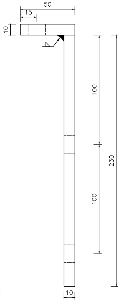
连接件侧面 (1:2)
