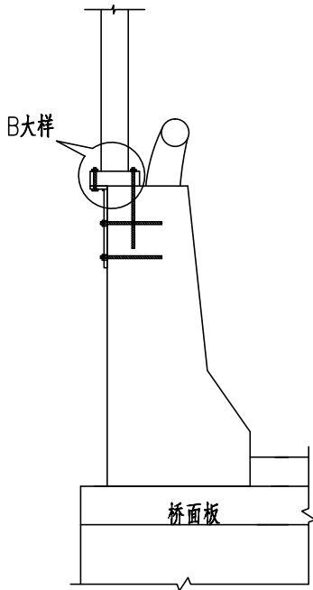
侧面图 (1:20)
