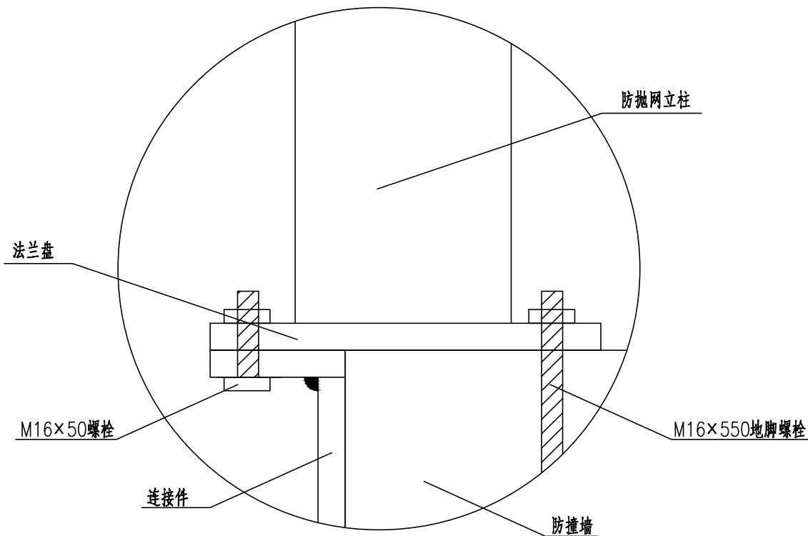
B大样
