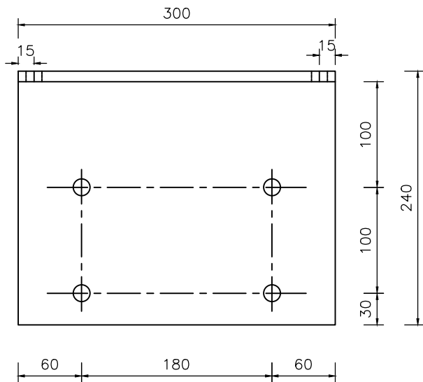
连接件正面 (1:5)
